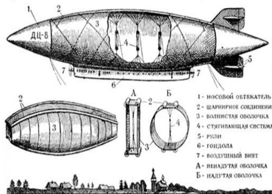
ЦЕЛЬНОМЕТАЛЛИЧЕСКИЙ ДИРИЖАБЛЬ ЦИОЛКОВСКОГО
